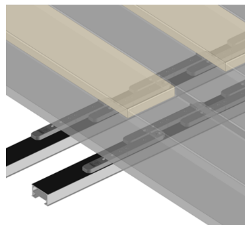
Double lambourdage
